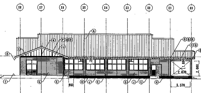
北側立面図 S=1:200
