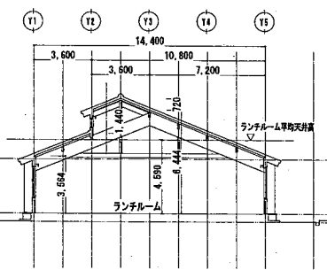
南-北断面図 S=1:200
