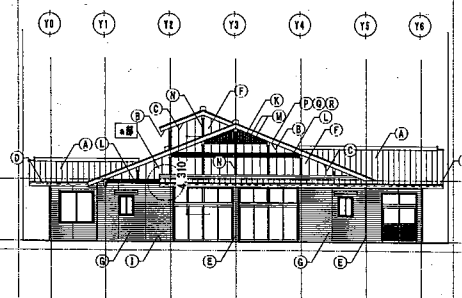
東側立面図 S=1:200
