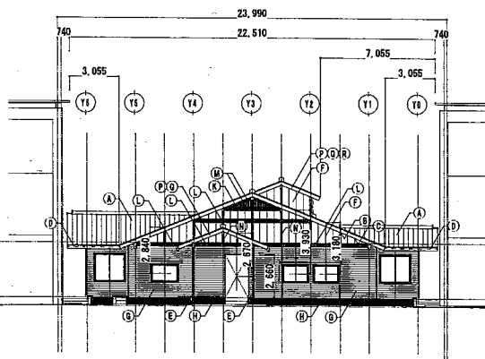
西側立面図 S=1:200
