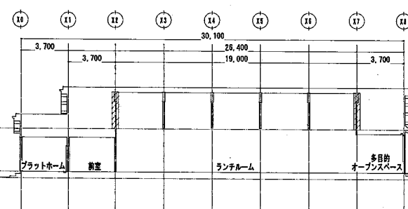
東-西断面図 S=1:200
