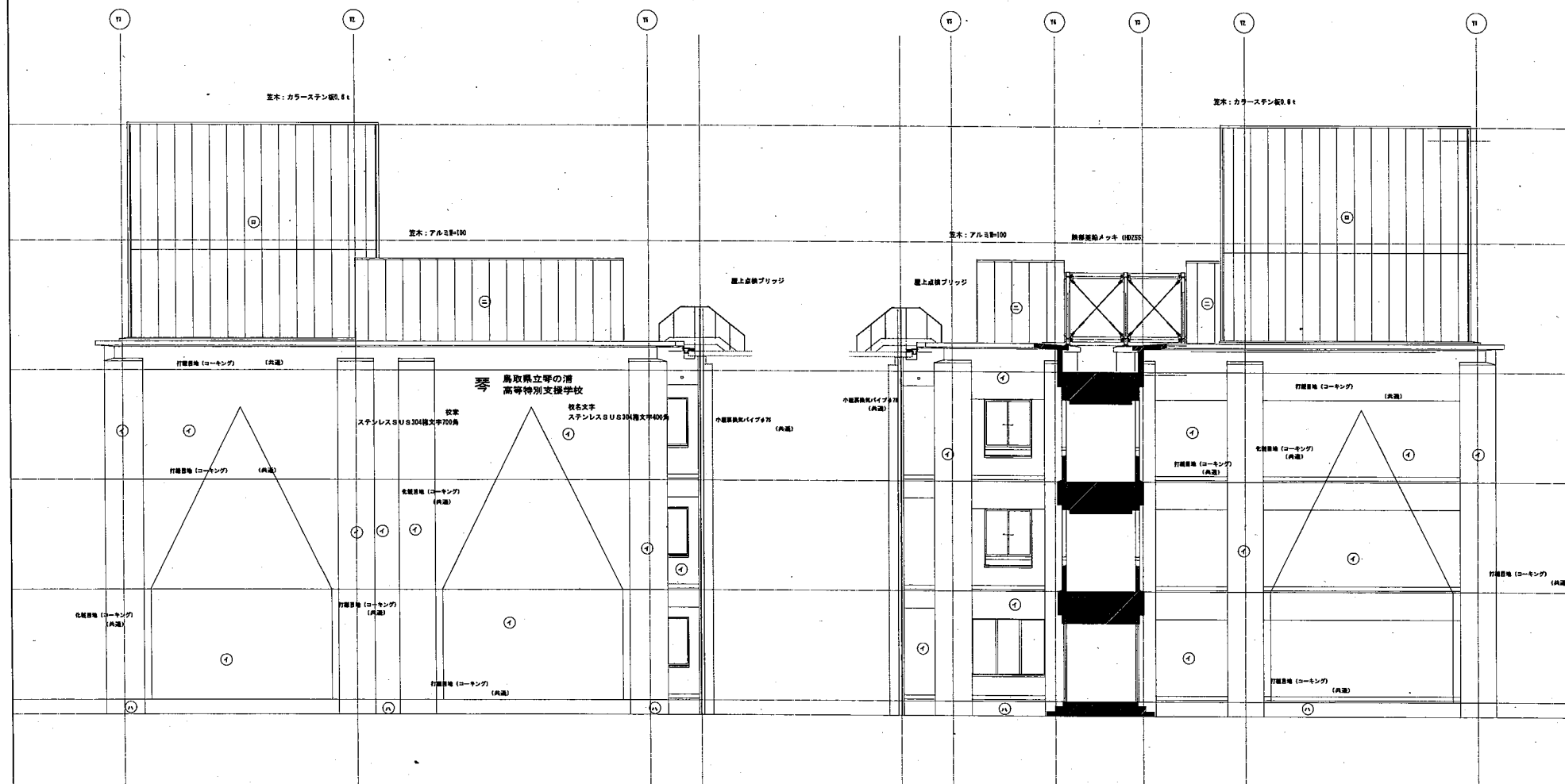
東面立面図
