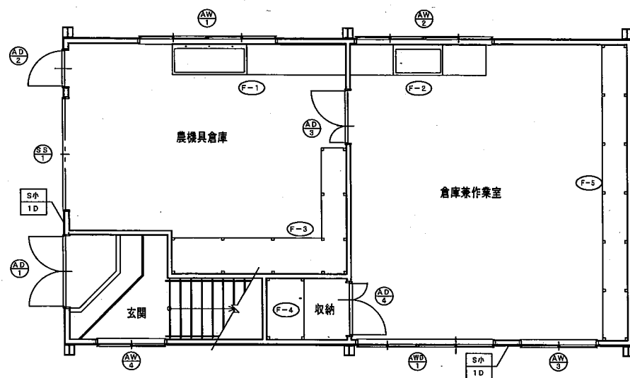
改修後1階器具配置図
