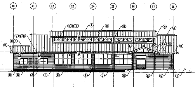
南側立面図 S=1:200
