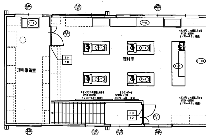
改修後2階器具配置図
