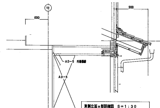
東側立面a部詳細図 S=1:30
