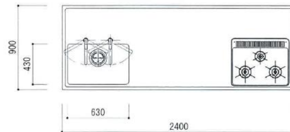
配管立上平面図
