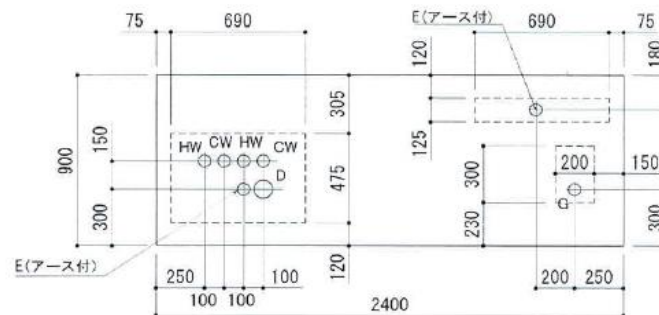
配管立上平面図
